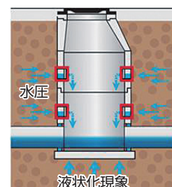
マンホールの浮上抑制対策
