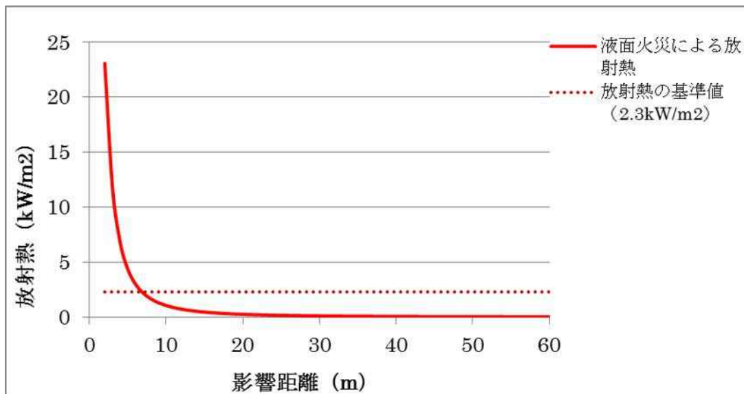
図3-1-2 液面火災の影響距離
