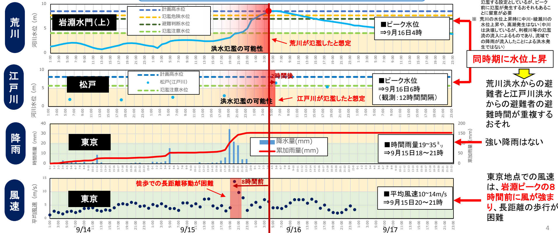
カスリーン台風における河川水位・潮位・降雨・風速の状況
