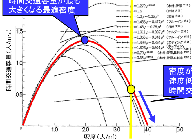
水平な通路における密度と時間交通容量※2
