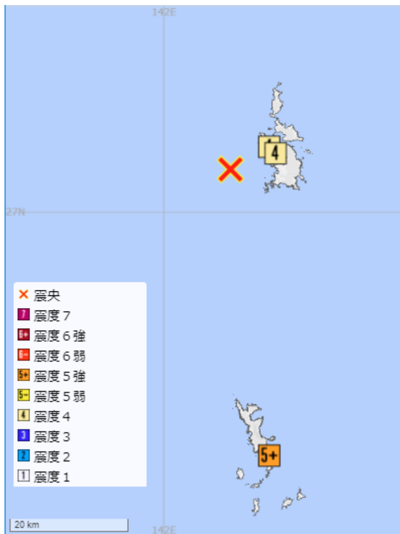
図 1 1 月 4 日 父島近海の地震の震度分布図
