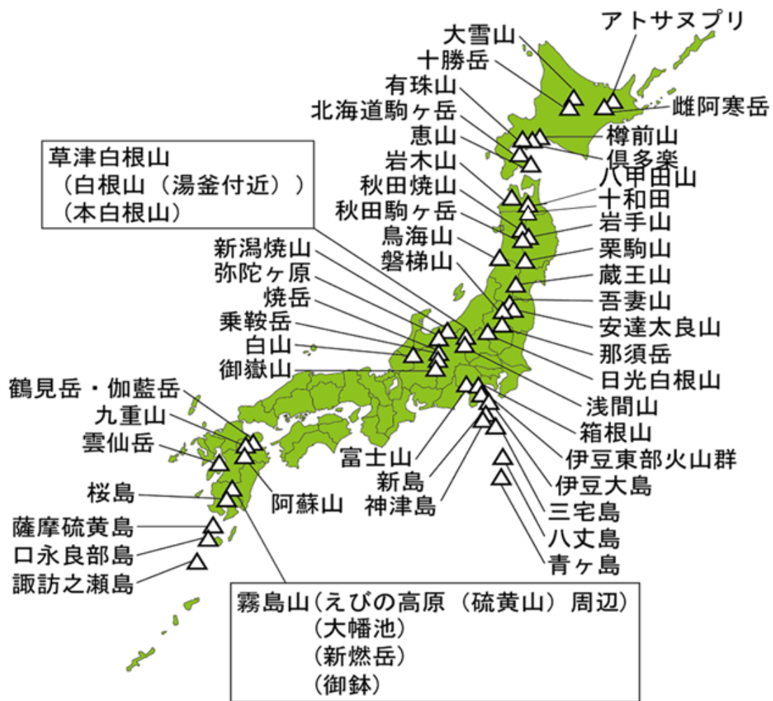
図2 噴火警戒レベルが運用されている火山 (令和4年12月時点)
