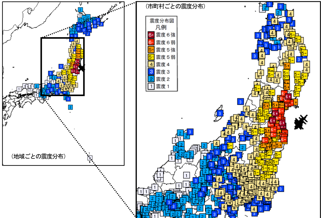
図2 3月16日 福島県沖の地震の震度分布図
