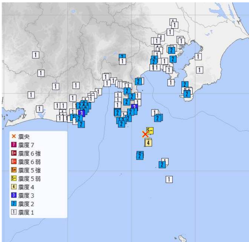
図3 5月22日16時42分 新島・神津島近海の地震の震度分布図
