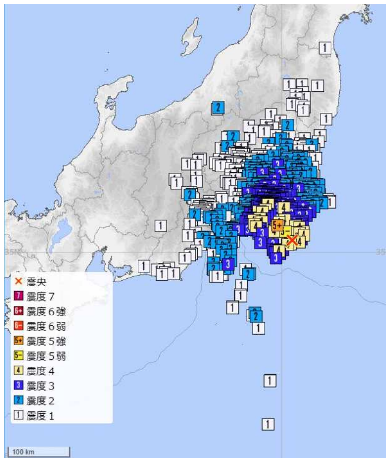
図2 5月11日 千葉県南部の地震の震度分布図
