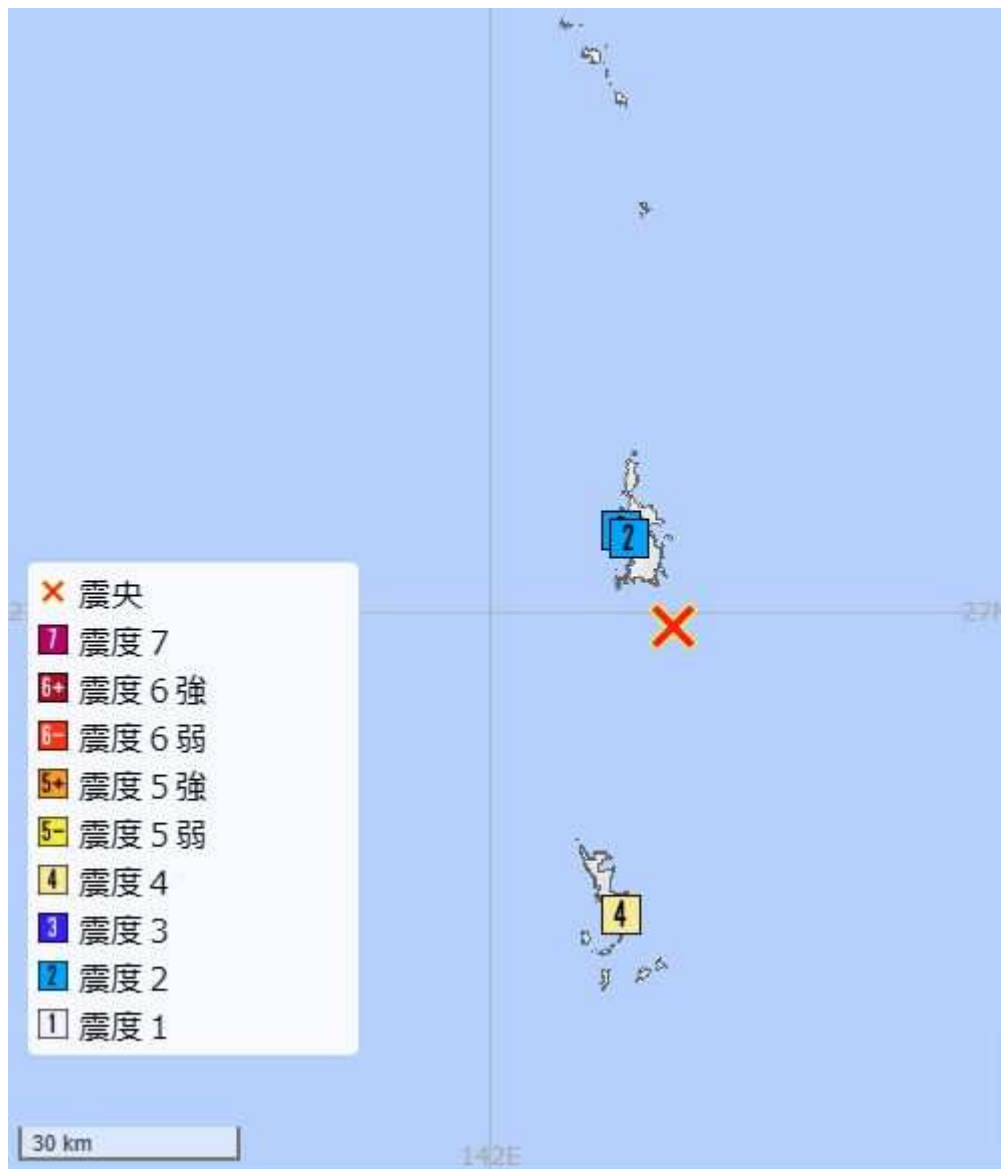
図1 4月21日 父島近海の地震の震度分布図
