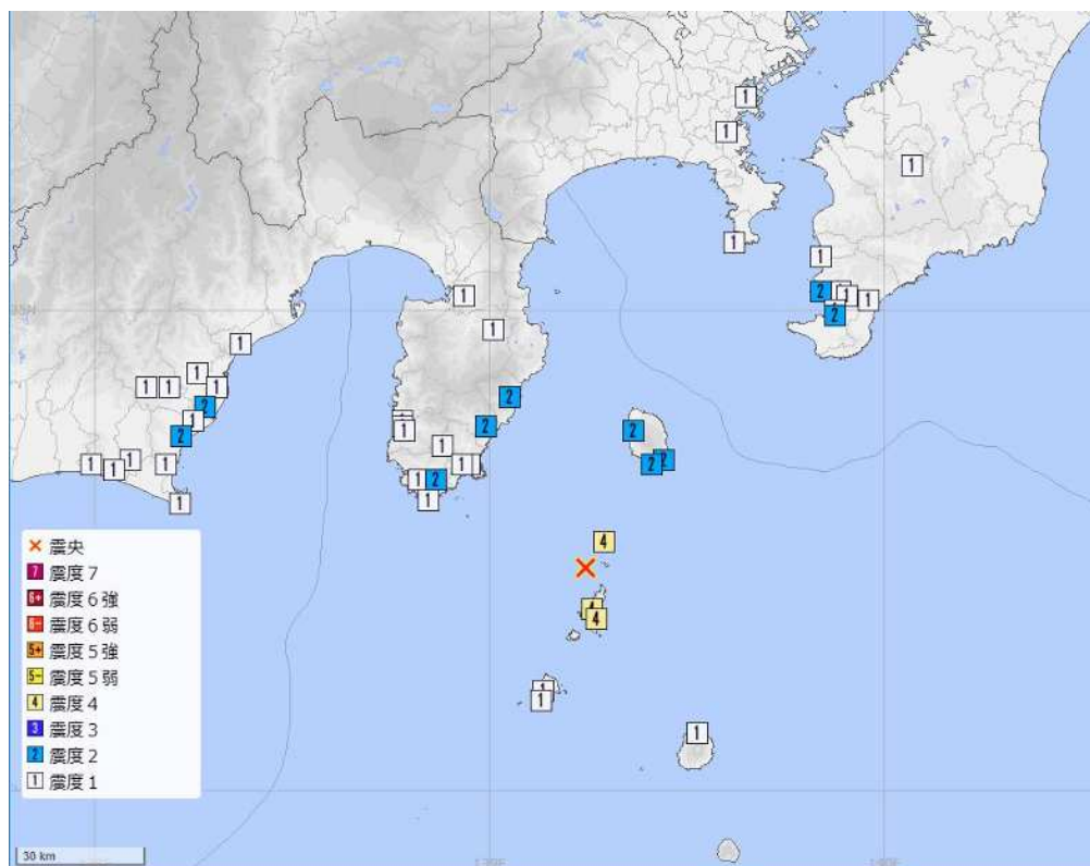
図4 5月22日19時46分 新島・神津島近海の地震の震度分布図
