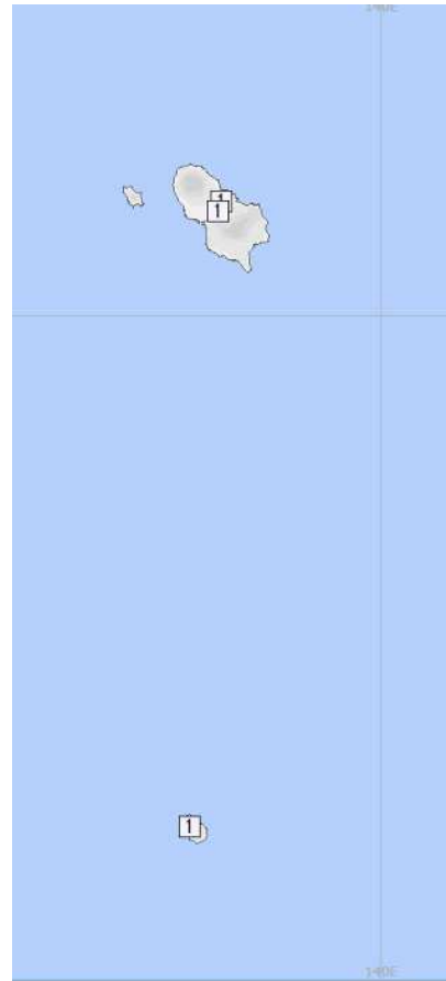
図3 5月22日16時42分 新島・神津島近海の地震の震度分布図
