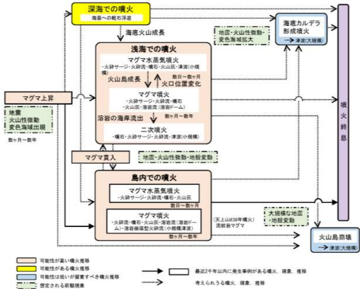
図 神津島火山の噴火事象系統樹
