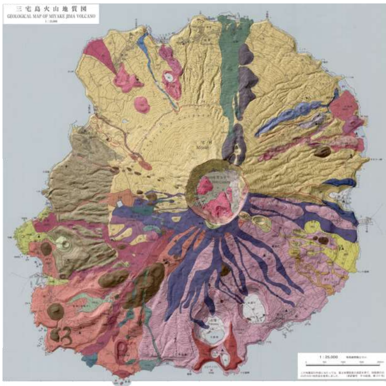
図 三宅島火山地質図(津久井ほか，2005)
