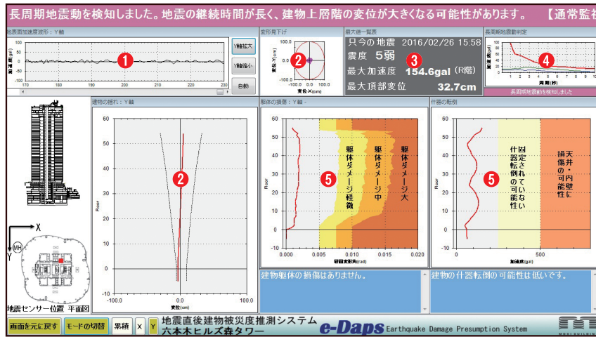
①地震計データの波形表示 ②建物の揺れをリアルタイム表示 ③地表面の最大加速度、建物内の最大加速度・最大変位、地表面震度の表示 ④長周期地震発生有無の表示 ⑤建物被災度推測解析(躯体損傷・什器転倒)の立面表示
