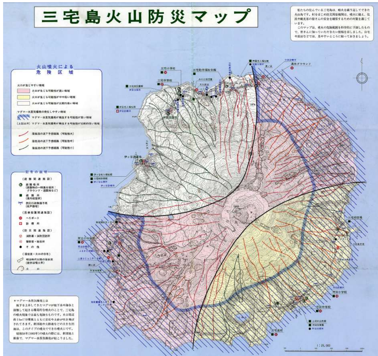
図 三宅島火山防災マップ(三宅村, 1994)
