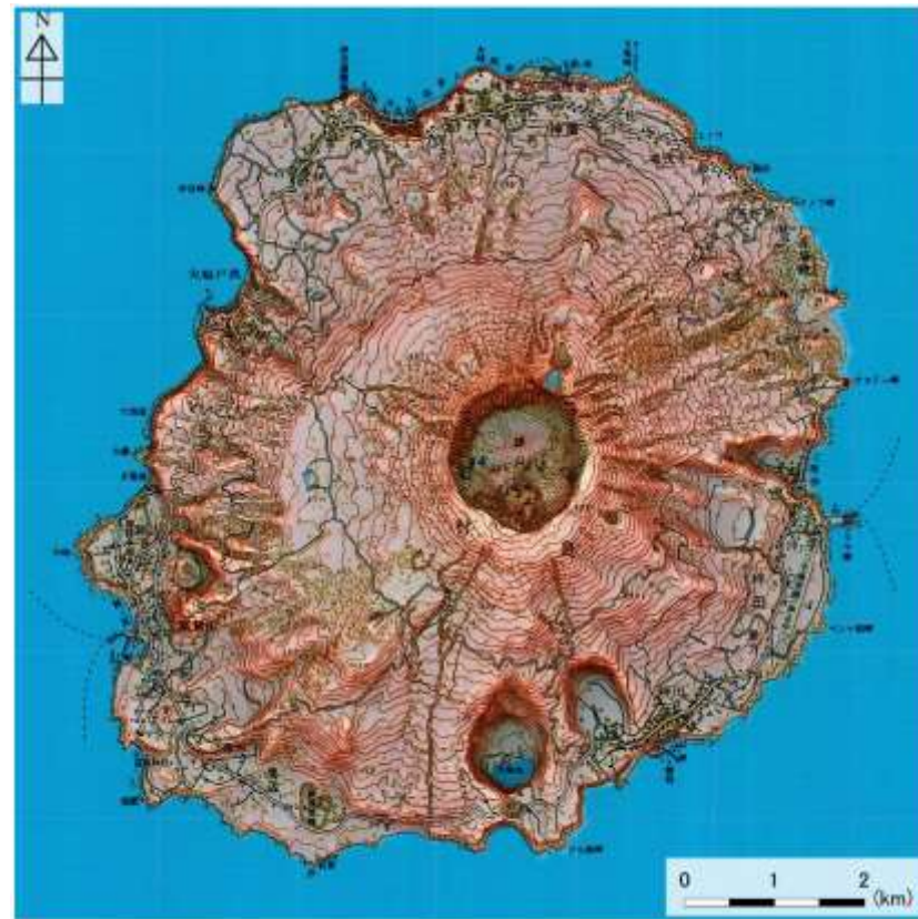
図 三宅島の地形図(気象庁, 2013)
