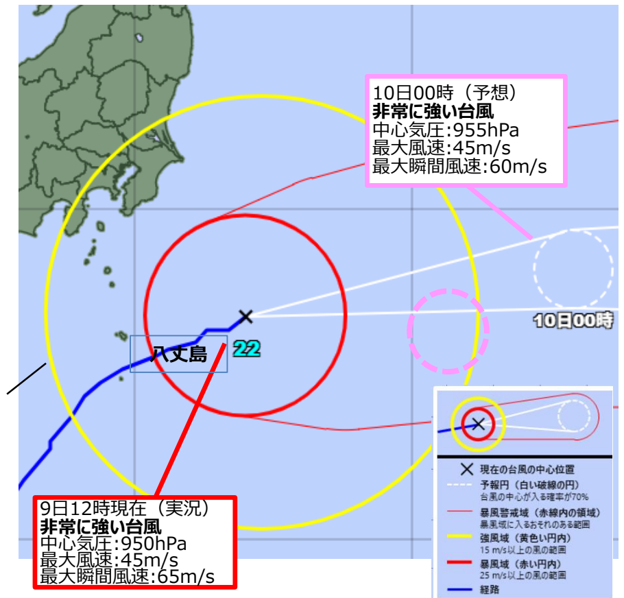
台風予想図 (9日12時時点)
