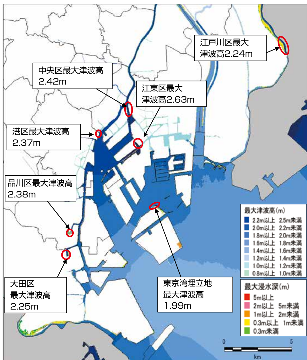
図 南海トラフ巨大地震（各メッシュにおける全5ケースの最大値）の各区における最大津波高とその場所
