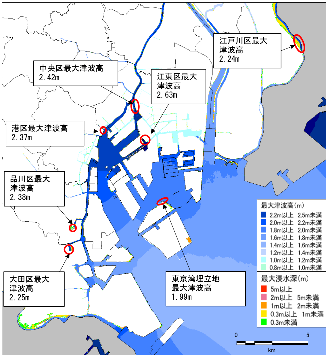
図 南海トラフ巨大地震（各メッシュにおける全5ケースの最大値）の各区における最大津波高とその場所
